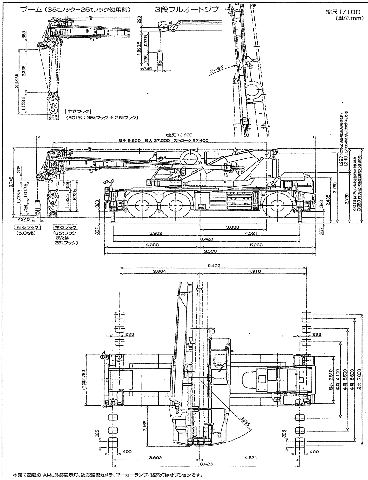
■主要寸法図
