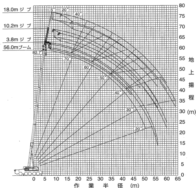
56.0mブーム+バイフォールドパワーチルトジブ
