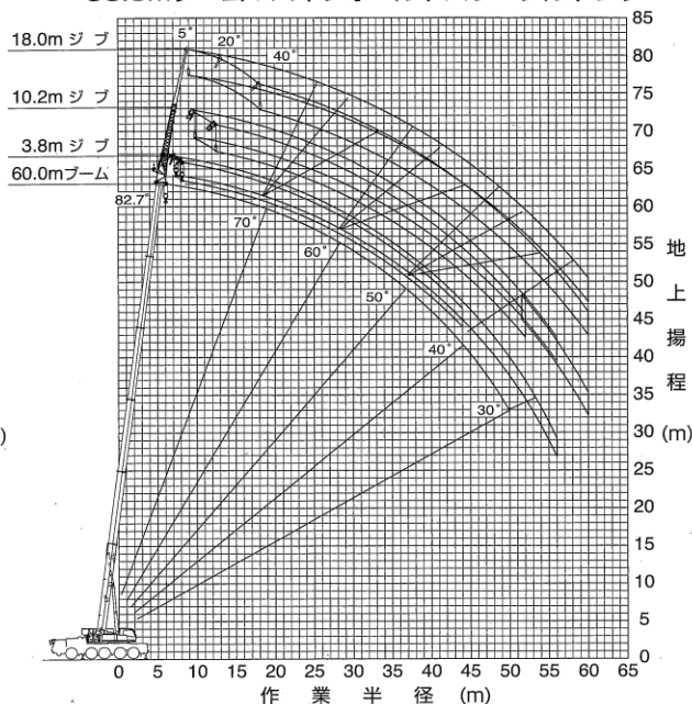
60.0mブーム+バイフォールドパワーチルトジブ
