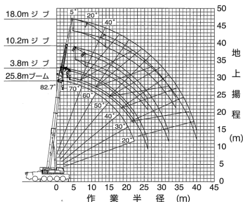
25.8mブーム+バイフォールドパワーチルトジブ
