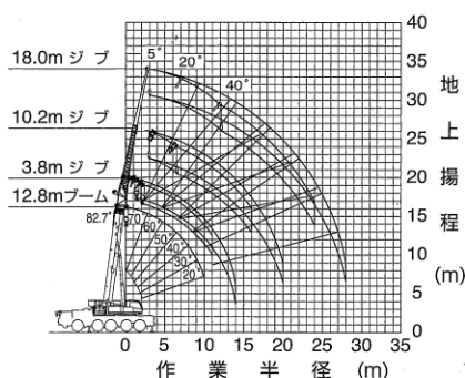
12.8mブーム+バイフォールドパワーチルトジブ
